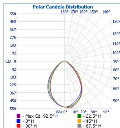
LZWET-1-UNV-840-11L-80-LD.ies
